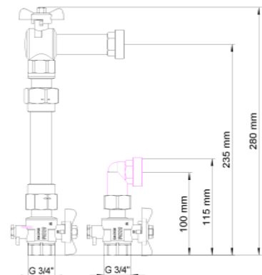
KM591E WMZ-Paßstück Winkel 90° 3/4"
