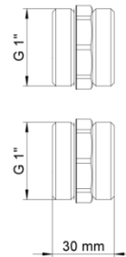
KM593E Anschluss Kugelhahn Winkel 90°
