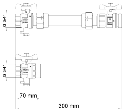
KM591E WMZ-Paßstück gerade 3/4"
