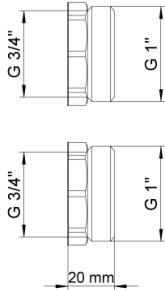
KM593E Anschluss Kugelhahn gerade
