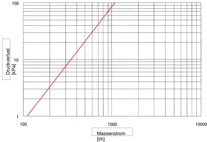
Diagramm der Durchflussmengenmesser im Vorlaufverteiler
